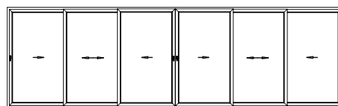
Schéma 3 ou 6 vantaux Dim. 3 vantaux : 4 x 2,6 m Dim. 6 vantaux : 5 x 2,6 m
